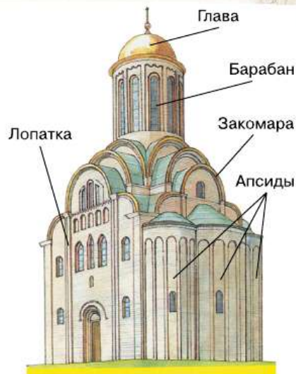
Церковь Параскевы Пятницы в Чернигове. Элементы крестово-купольного храма
